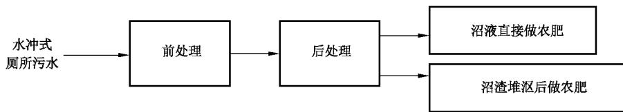
图 B.2 无管网水冲式厕所沼气净化池处理工艺流程
